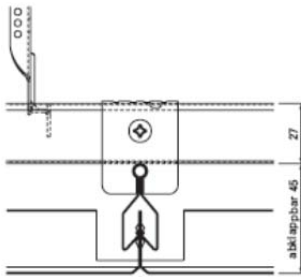
Detailschnitt
