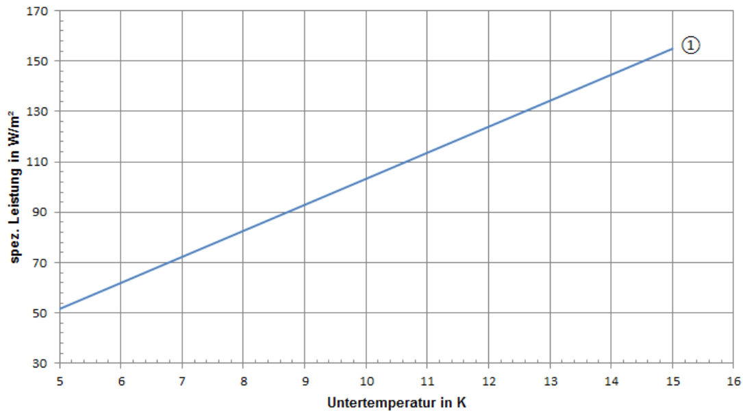
spezifische Kühlleistung
