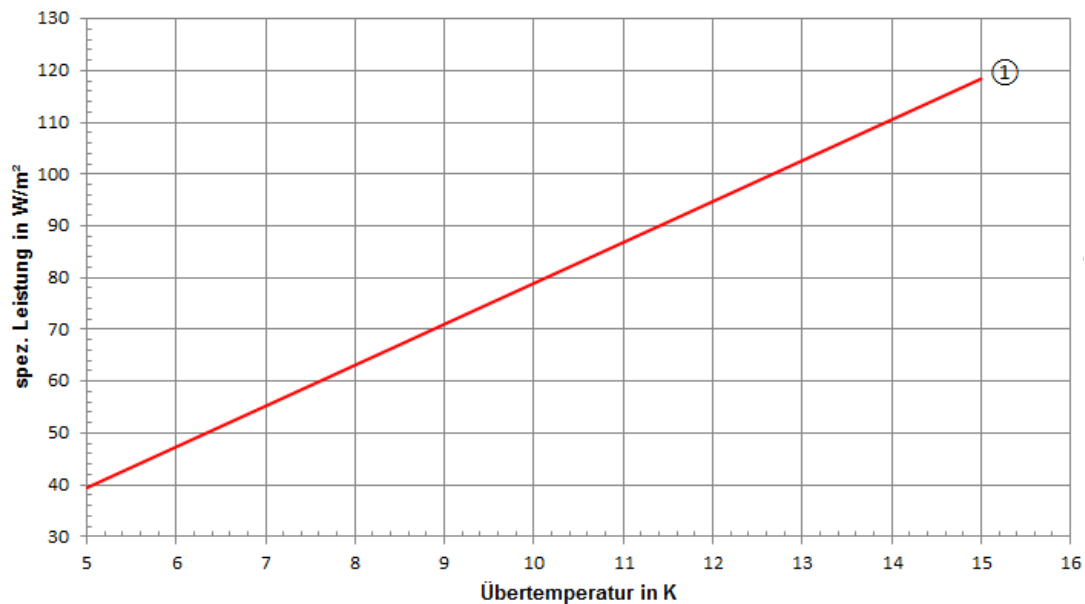
spezifische Heizleistung
