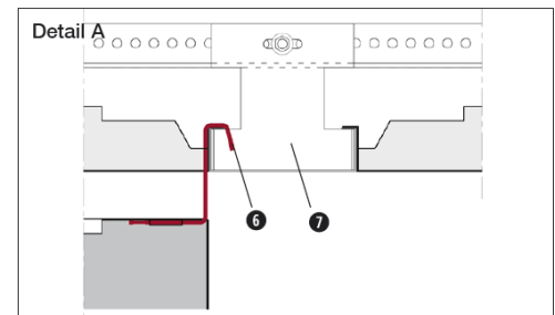
DOOR-Bügel für Abklappfunktion (Bügelstärke und Ausführung abhängig vom Kassettengewicht)
