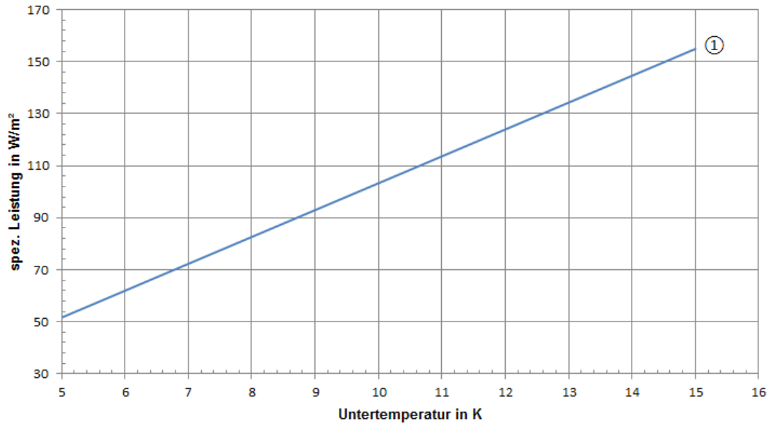
spezifische Kühlleistung
