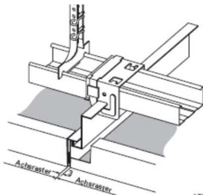
Detailschnitt
